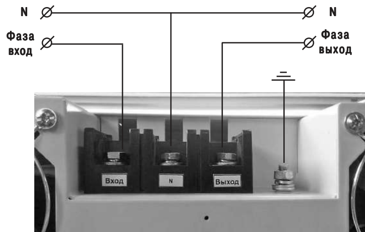
Рис. 4. Схема подключения стабилизатора
