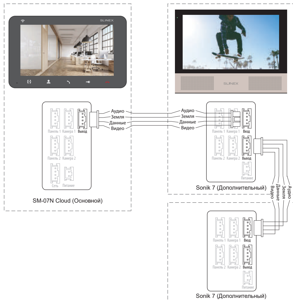
Схема 2. Подключение системы домофонов SM-07N Cloud и Sonik 7.
